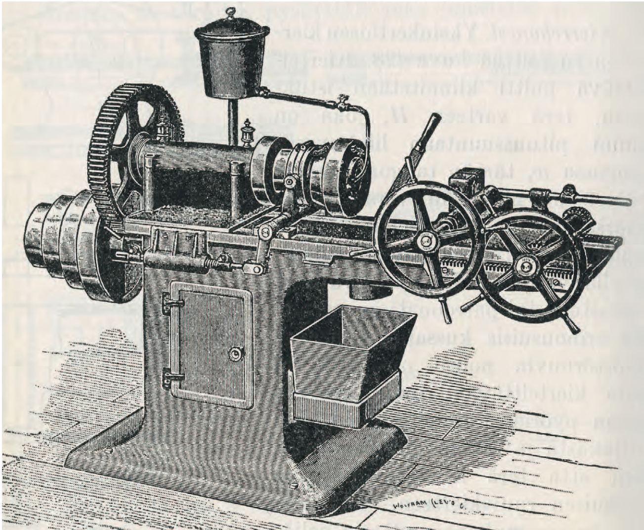
Paavo Peron teos oli yksi tärkeä avain tekniikan maailmaan. Kuvassa pulttikierrekone kyseisestä kirjasta.
